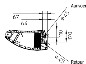
Aanzuigzijde
