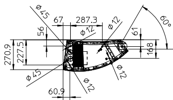
Vloerconsole
