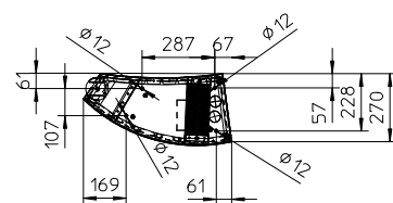
Vloerconsole
