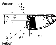
Onderaansluitingen
