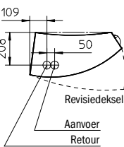
Bovenaansluitingen
