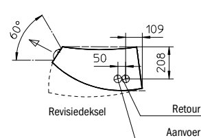
Bovenaansluitingen
